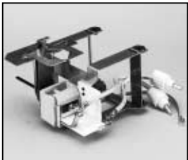
L4.79123.E Lamp holder + lamp carriage (refurbished) only as Exchange-Part available! Lampenfassung und Fassungsträger Nur aus Austausch-Teil verfügbar !
